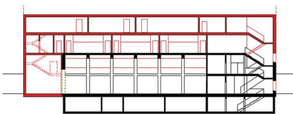
Längsschnitt 1:500
