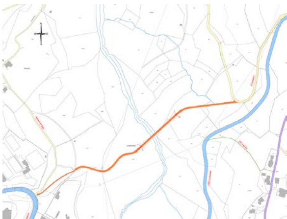
Auszug aus dem Entwurf des Teilstrassenplans mit dem Verlauf der Zugänge und der Fuss- und Velowegbrücke St. Gallen-Untereggen
